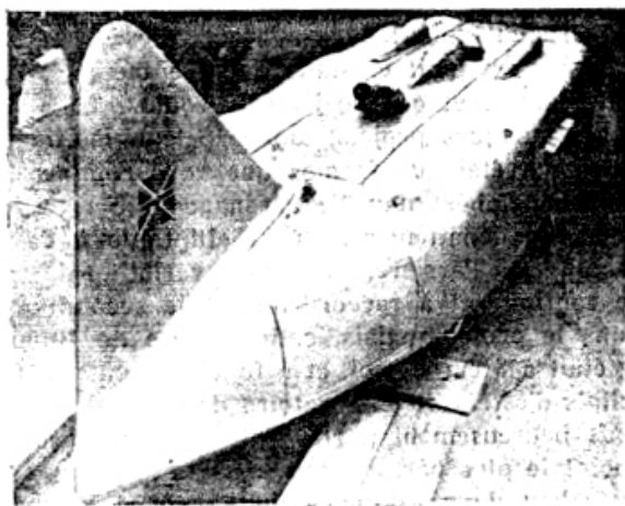
On remarque sur cette photographie les entrées d'air pour les carburateurs et le refroidissement, l'habitacle de tête, les tuyaux d'échappement et les sorties d'air.
